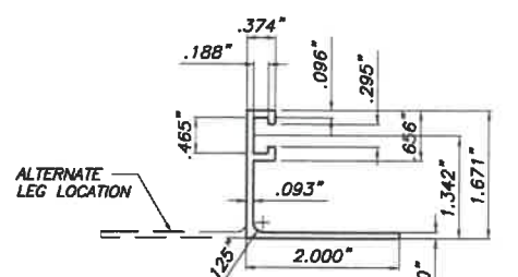
8 'F' TRACK ANGLE SCALE: 3/8" = 1"
